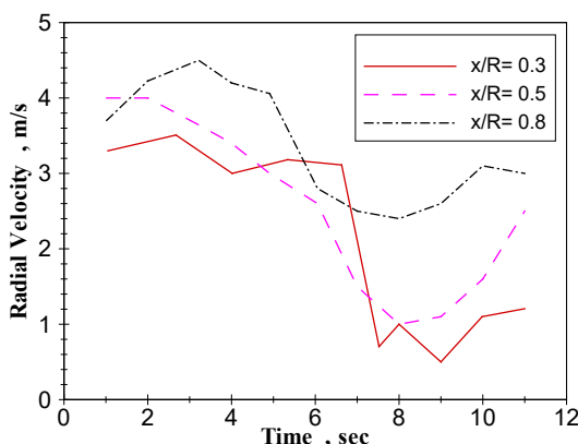
شکل ۱- تغییرات سرعت شعاعی نسبت به زمان (فونت: BZar, اندازه فونت ۹ ضخیم)
